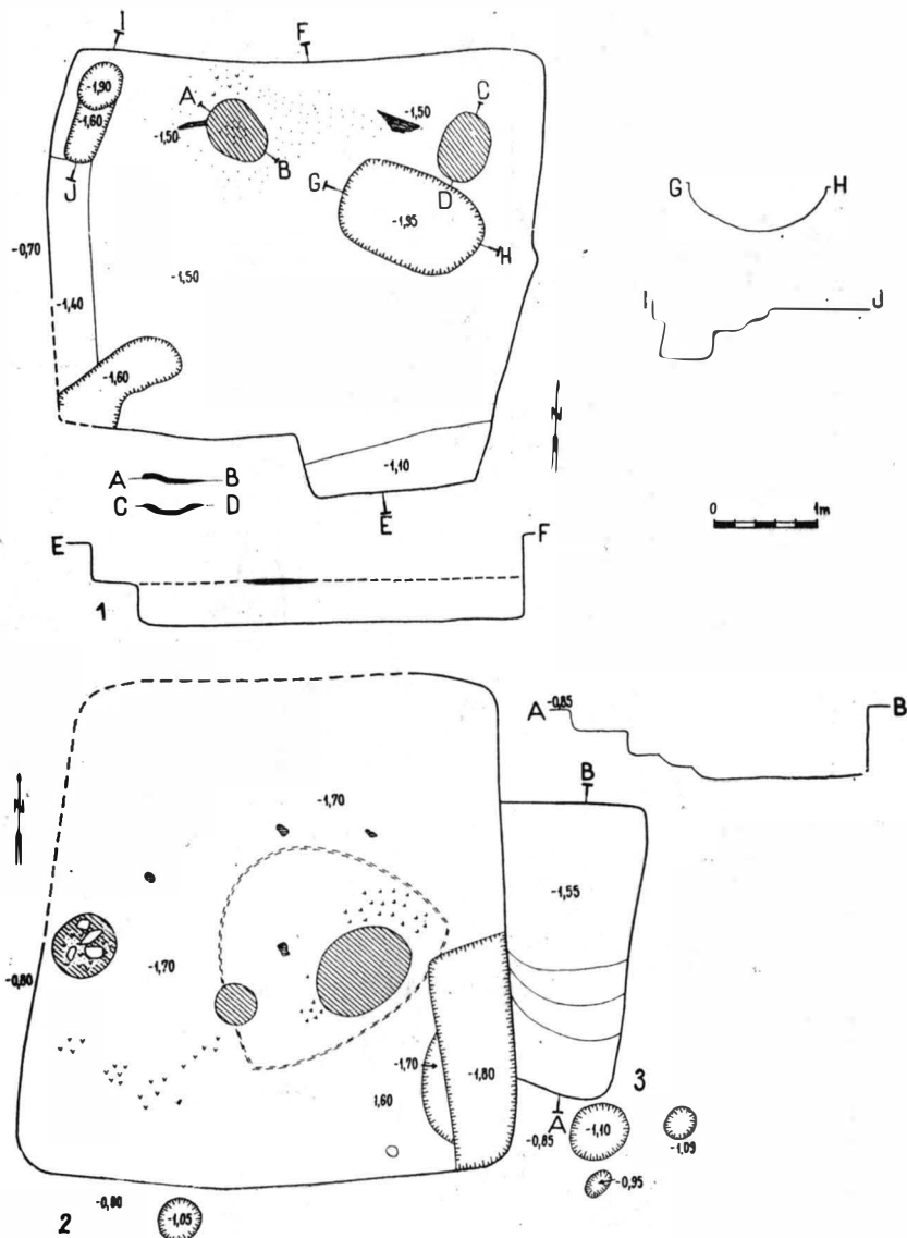
Fig. 10 Bucov-Tioca. 1 planul și profilurile bordeiului 19; 2 planul bordeiului 21; 3 planul bordeiului 22.
