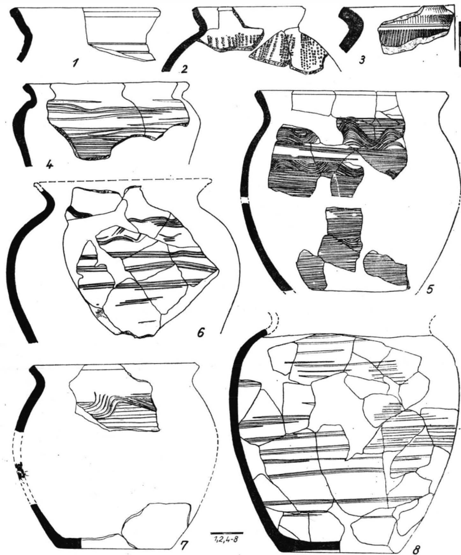
Fig. 71 Ceramică lucrată pe roata de mină, secolul X. Bucov-Tioca, casa 2.
