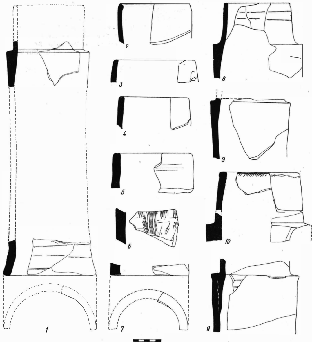
Fig. 28 Diferite tipuri de olane din pastă fină roz sau alburie. Bucov-Rotari. 1, 2, 8 bordeiul 1; 3, 4, 11 groapa de acces a cuptorului de pline; 6 casa 3; 7 casa 8; 9 dependența 4; 10 casa 9; Bucov-Tioca. 5 secțiunea 3, caroul 7.
