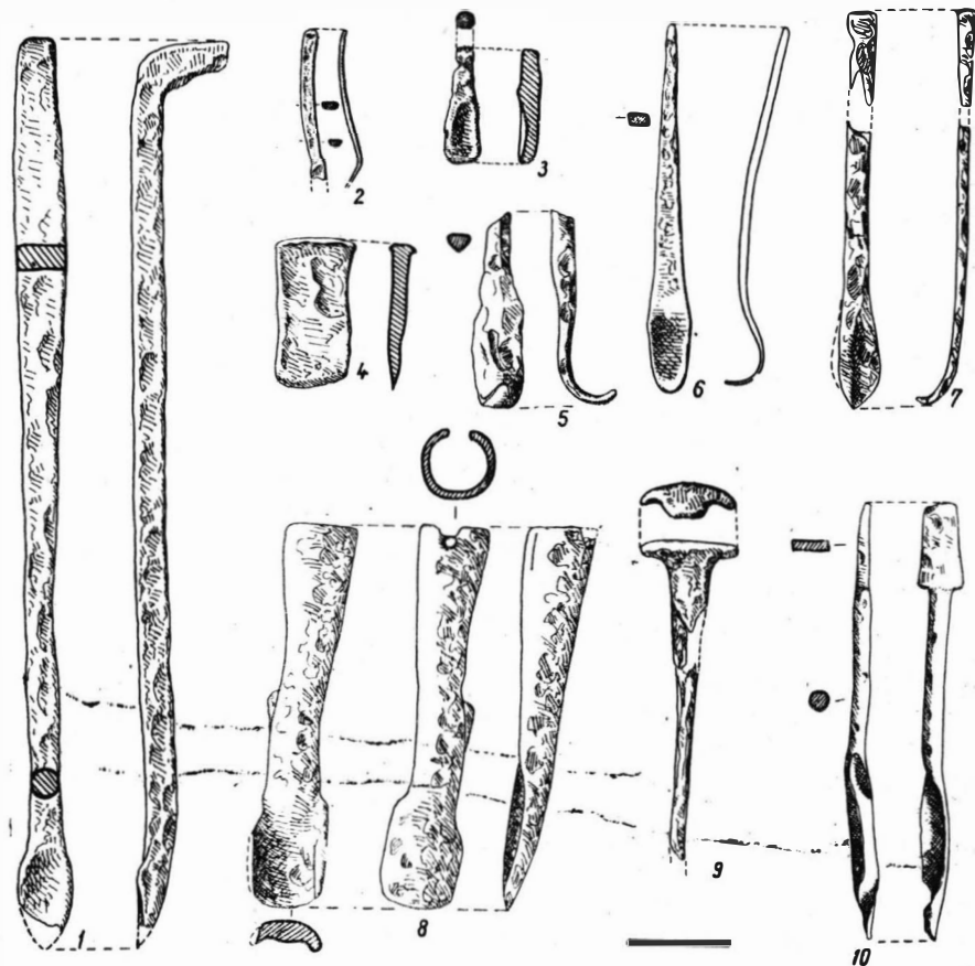
Fig. 35 Unelte pentru prelucrarea lemnului. 1 Bucov-Rotari, în apropierea laturii de sud a dependinței nr. 2; 2, 4 Bucov-Rotari, casa 2; 3 Bucov-Tioca, bordeiul 2; 5, 7 Bucov-Tioca, casa 6; 6 Bucov-Tioca, casa 17; 8 Bucov-Tioca, în apropierea laturii de est a casei 12; 9 Bucov-Tioca, bordeiul 3; Bucov-Rotari. 10 casa nr. 3.
