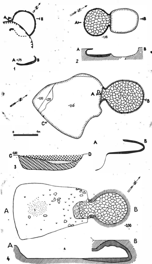
Fig. 27 Bucov-Tioca. 1 planul și profilul păstrat al cuptorului 2; 2 planul și profilul cuptorului 1; 3 planul și profilul cuptorului 4 și al gropii de acces al acestuia. Bucov-Rotari. 4 planul și profilul cuptorului de copt.
