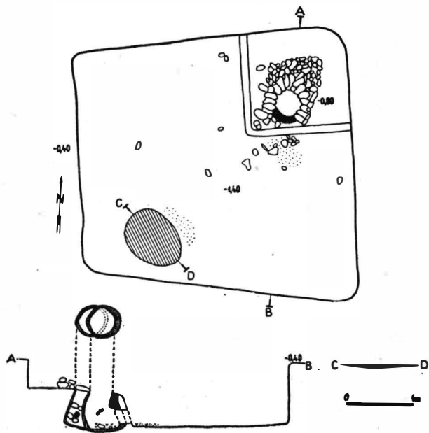
Fig. 32 Bucov-Tioca. Planul bordeiului-atelier nr. 5 și profilul său, indicînd cele două faze de existență ale cuptorului pentru redus minereul de fier (vezi legenda la fig. 6).
