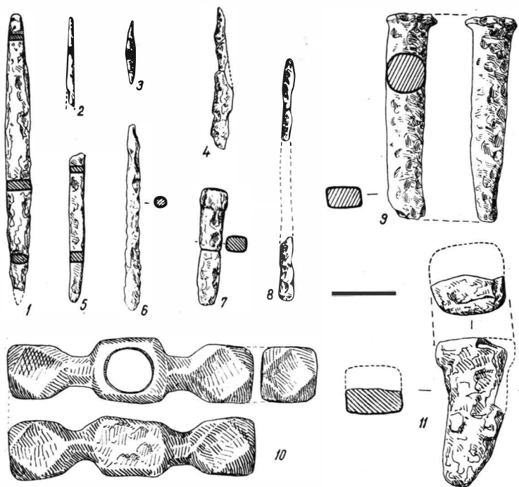
Fig. 34 Unelte pentru prelucrarea fierului (1-8 pile; 9, 11 nicovală; 10 ciocan). 1 Bucov-Rotari, depindeința nr. 2 (atelier de fierărie); 2-3 Bucov-Tioca, casa 11 (atelier de fierărie); 4 Bucov-Tioca, bordeiul 4; 5 Bucov-Rotari, depindeința 4 (atelier de fierărie); Bucov-Rotari. 6 depindeința nr. 3; 7 depindeința nr. 2 (atelierul de fierărie); 8 Bucov-Tioca, casa 12; 9, 11 Bucov-Tioca, bordeiul 12; 10 Bucov-Rotari, în preajma depindeinței nr. 2 (atelierul de fierărie).
