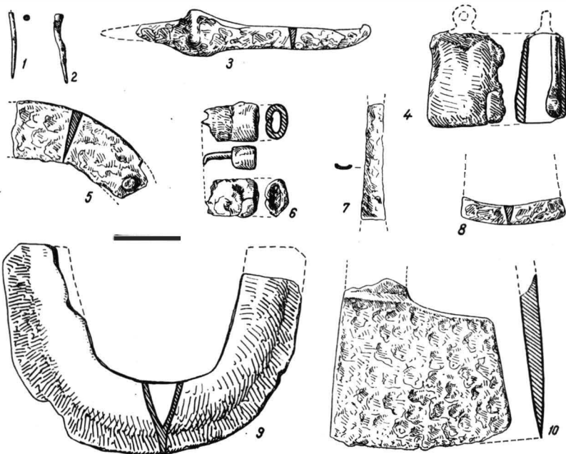
Fig. 30 Diferite unelte de fier. Bucov-Tioca. 1 casa 11, sulă sau ac; 2 casa 12, sulă (?); 3 bordeiul 9, cuțit pentru tăiatul pieilor; 4 casa 10, talangă; 5 bordeiul 16; 6 casa 6a, tindeică pentru întins plinza; 8 casa 11, fragment de topor; 9 casa 6, ramă de hrlleț; Bucov-Rotari. 7 casa 3; 10 casa 9, fragment de topor.
