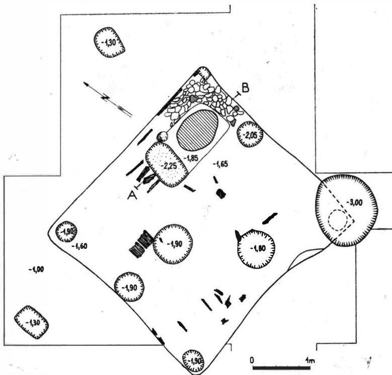
Fig. 7 Bucov-Tioca. Planul bordeiului 6 și profilul celor două vetre adâncite (fiecare avînd cite o refacere). 1 pămînt cenușiu închis din umplutura gropii bordeiului. 2 pămînt cenușiu, conținînd lentile de pămînt ars, roșu-vinețiu, din umplutura gropii-cenușar din fața vetrelor și de pe ultima vatră; 3 pietre care căptușiseră peretele în dreptul vetrei, căzute peste ultima vatră și în groapa cenușar; 4 arsura vetrei; 5 pămînt galben adus special și așezat peste prima vatră pentru a servi ca postament pentru vatra a doua; 6 cenușă; 7 cărbuni.
