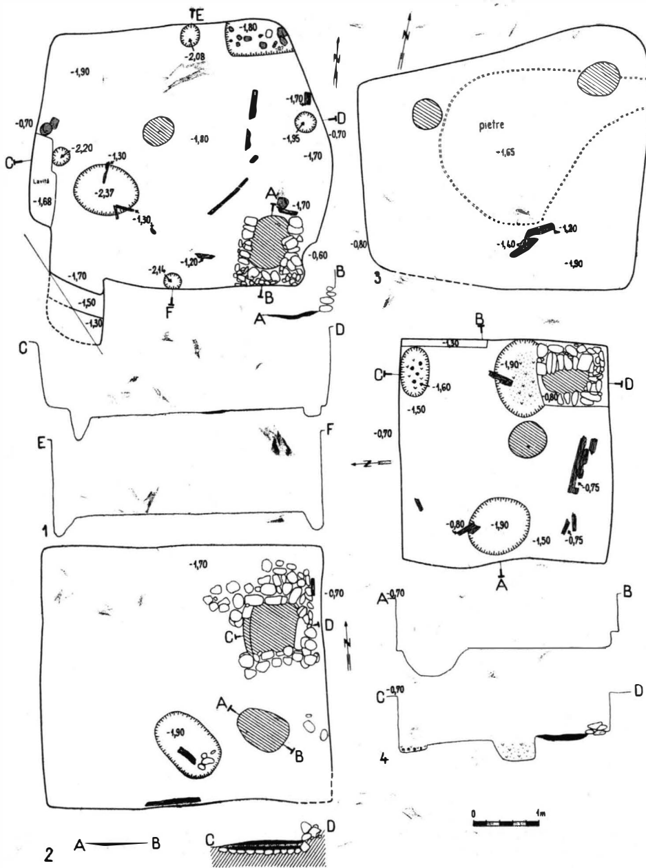
Fig. 11 Bucov-Tioca. 1 planul și profilurile bordeiului 17; 2 planul și profilul vetrelor bordeiului 18; 3 planul bordeiului 20; 4 planul bordeiului 23.
