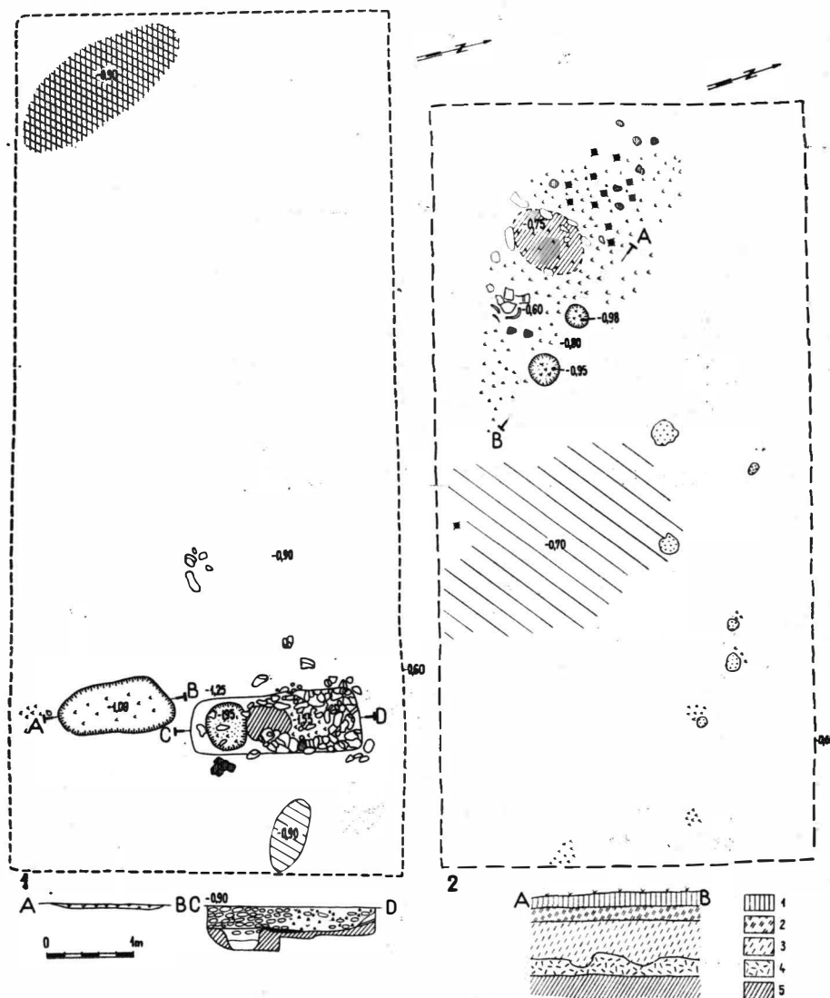
Fig. 23 Bucov-Rotari . 1 planul casei 1 și profilul vetrei adîncite în groapă din interiorul ei; 2 planul casei 2 (1 humus; 2 pămînt cenușiu cafeniu corespunzător epocii feudalismului dezvoltat; 3 pămînt cenușiu-cafeniu cu resturi arheologice din epoca feudală timpurie; 4 pămînt cenușiu-gălbui cu resturi din epoca hallstatiană; 5 pămînt viu).
