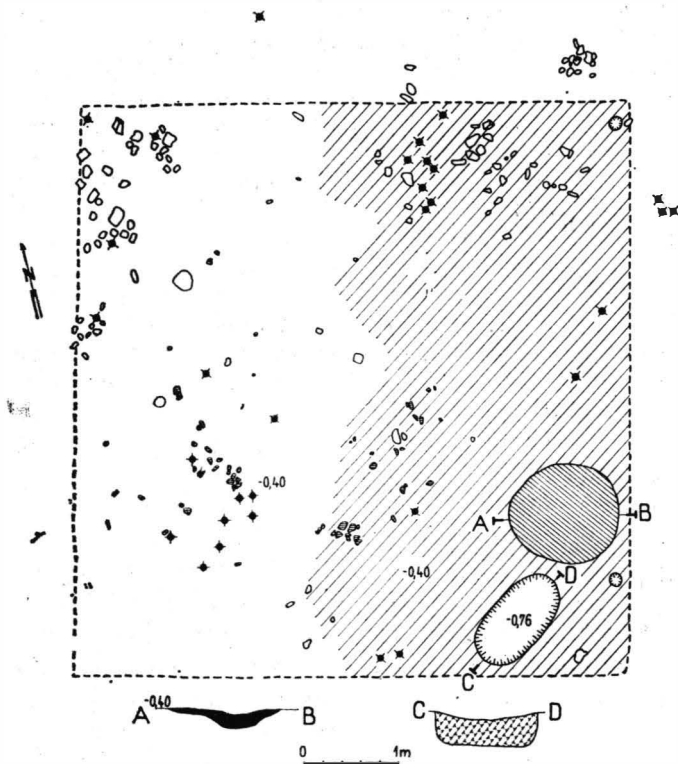
Fig. 33 Bucov-Tioca. Planul casei 11, în care se afla și un atelier de fierărie.
