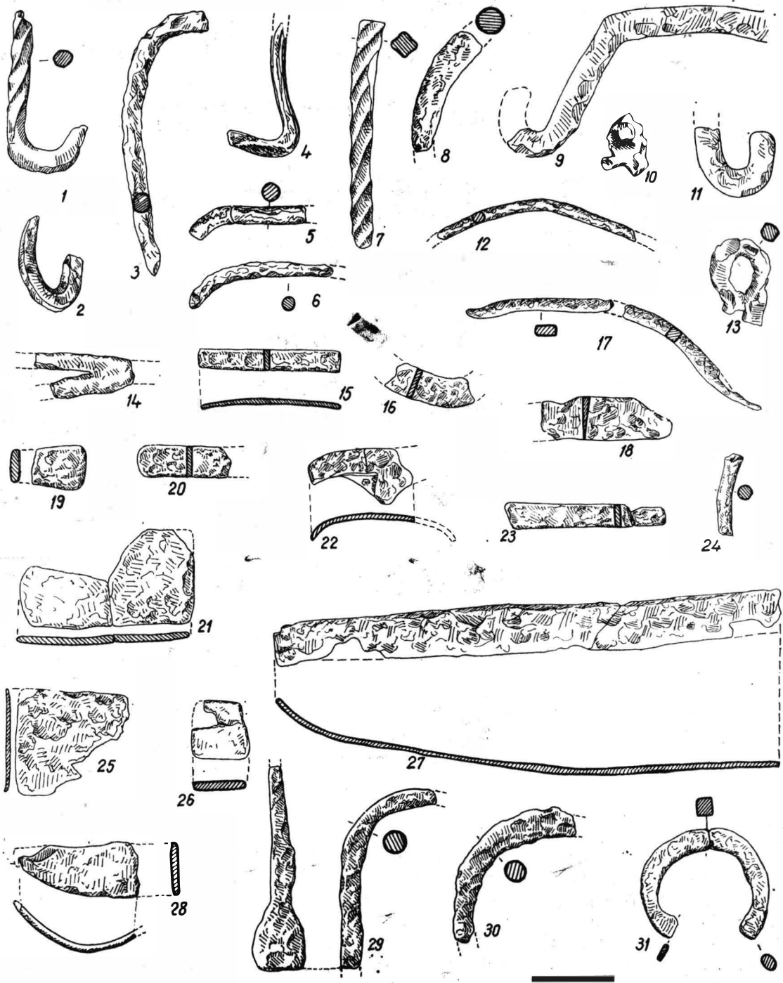
Fig. 93 Fragmente de toarle și de cercuri, diferite ornamente de fier de la găleși de lemn. Bucov-Rotari. 1 casa 6; 3 casa 4; 10, 13 dependința nr. 2; 24 dependința nr. 5 (atelier de fierărie); 26 secțiunea „R”, caroul 10, -0,70 m (în nivelul de locuire al bordeiilor). Bucov-Tioca. 2, 18 casa 1; 5, 25 bordeiul 3; 6 secțiunea IV, caroul 4, -0,40 m (nivelul de locuire al caselor adâncite); 7-9, 11, 31 casa 14; 12 casa 7; 14, 19, 20, 21 bordeiul 2; 15 bordeiul 9; 16, 22 casa 11; 17 casa 12; 18 casa 1; 27 groapa nr. 2; 28 bordeiul 9; 29, 30 casa 17.
