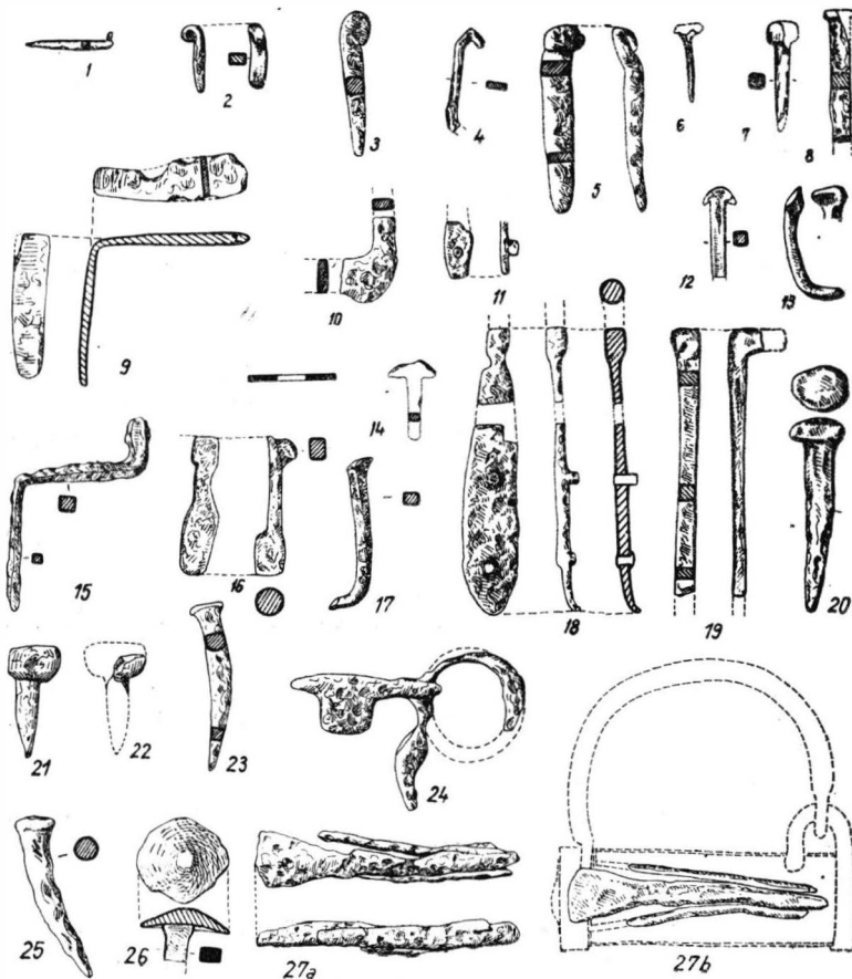
Fig. 26 Diferite obiecte: cuie, cheie (24) și lacăt (27 a, b) de fier. Bucov-Rotari. 1 casa 1; 2 casa 5; 4 dependența nr. 2 (atelier de fierărie); 7, 9, 15 dependența nr. 3; 8 casa 6; 20 dependența nr. 5; 23, 25 casa 9. Bucov-Tioca. 3 bordeiul 9; 5 bordeiul 16; 6 casa 7; 10 bordeiul 7; 11, 16 bordeiul 3; 12, 13 casa 4; 14 bordeiul 19; 17 bordeiul 16; 18 casa 1; 19 casa nr. 25; 21 casa 4 c; 22 bordeiul 9; 24, 26 casa 11 (atelier de fierărie); 27 a-b casa 17.
