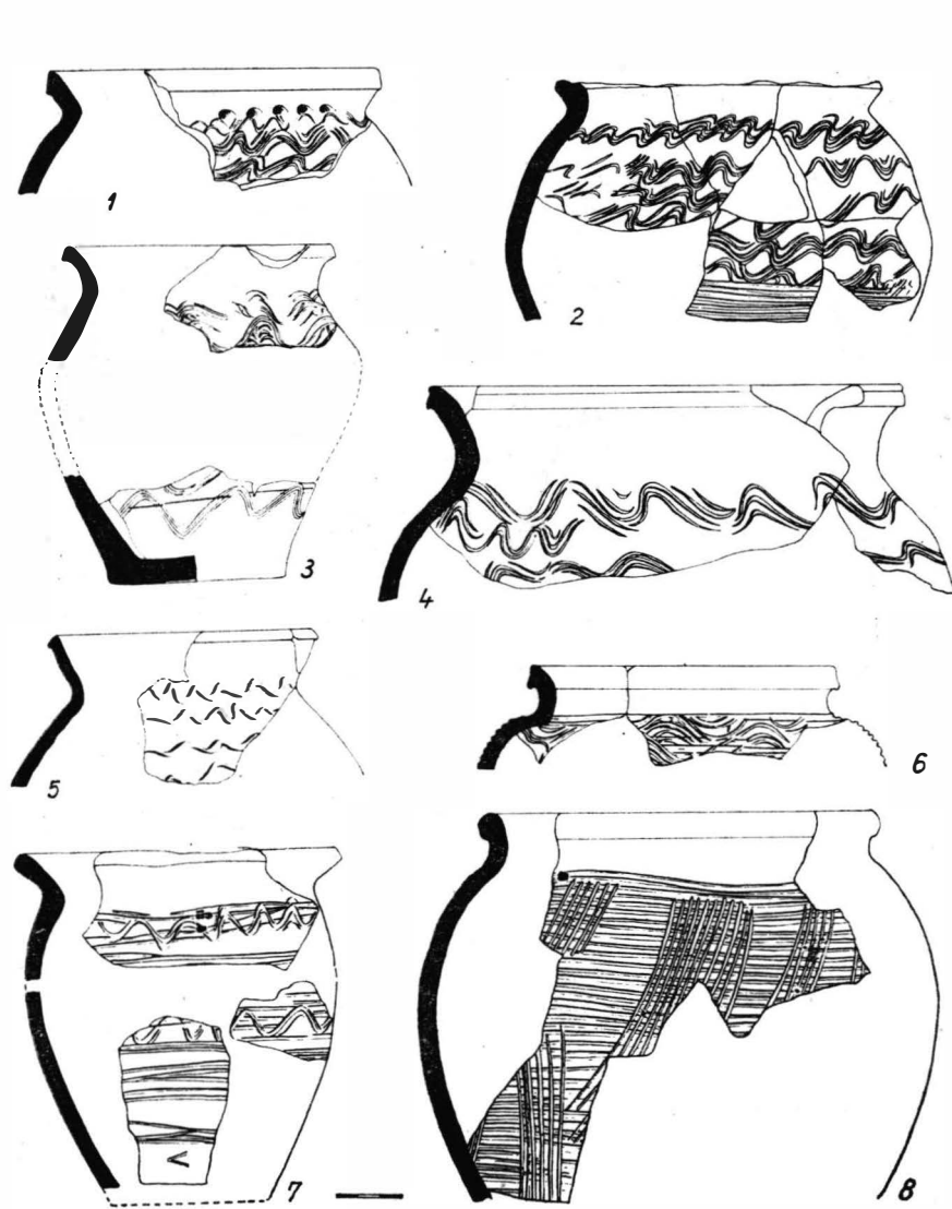
Fig. 63 Ceramică lucrată pe roata de mină din a doua jumătate a secolului IX și începutul secolului X. Bucov-Tioca, casa 12.
